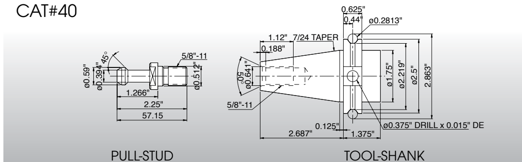
DIN#40 69871/72
